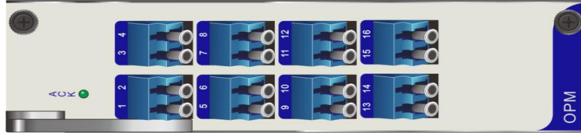
16 路 OPM 功率计板卡
