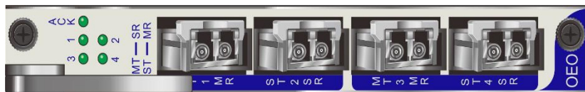
4路互环板卡
